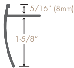
CM4050
